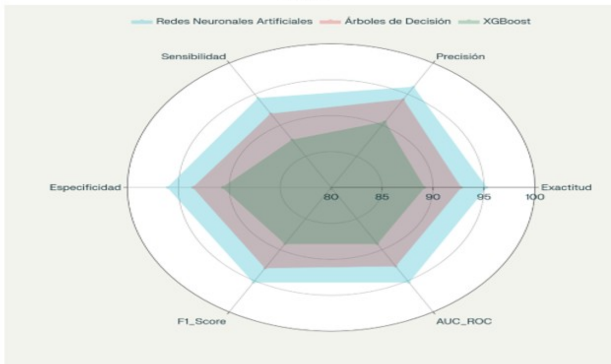
Gráfico 2. Perfil comparativo de métricas de rendimiento de los tres mejores algoritmos de machine learning
