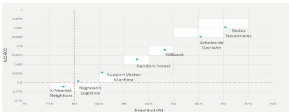
Gráfico 3. Correlación entre exactitud y AUC-ROC de algoritmos de machine learning para predicción de fracaso terapéutico en tuberculosis
